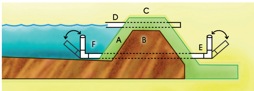
Figura 12. Corte sagital del borde de drenaje. A: borde con inclinación para evitar deslizamientos, B: corazón de arcilla, C: terraplén, D: tubo de rebose para evitar derrames en temporada de lluvias, E: tubo de drenaje externo con capacidad de inclinarse para ajustar el nivel de vaciado del estanque, F: tubo de drenaje interno con capacidad de inclinarse para ajustar el nivel de vaciado del estanque.
