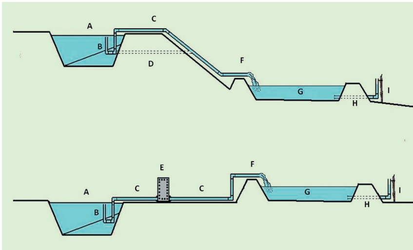
Figura 13. Croquis simplificado del sistema de llenado y drenaje de estanques en terreno con pendiente y a nivel.
