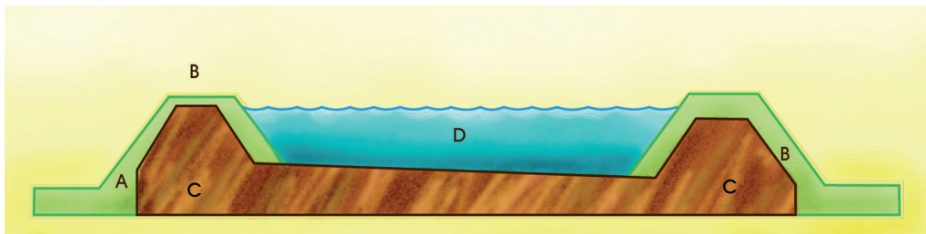
Figura 11. Corte sagital de un estanque de producción. A: borde para instalación de sistema de llenado, B: borde para instalación de sistema de drenaje, C: corazón de arcilla para incrementar la impermeabilidad del estanque, D: pendiente en el fondo para hacer más eficiente el drenaje parcial o total del estanque, E: terraplenes para el mantenimiento del estanque o manejo del cultivo.
